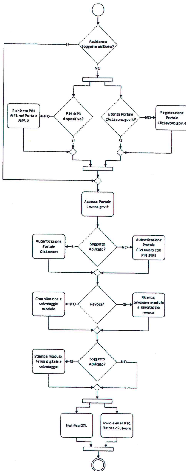
Figura 1 – Diagramma di flusso Invio Recesso Rapporto di Lavoro
